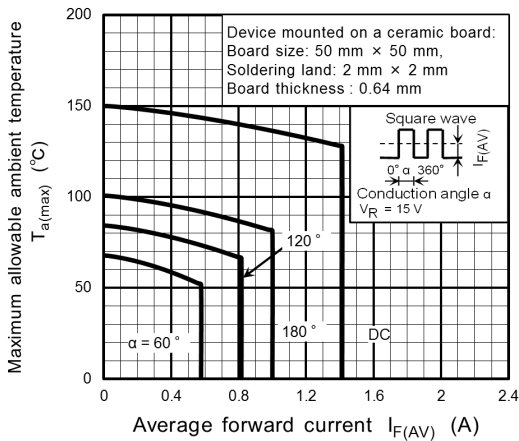
Fig. 10.3 T_{a(max)} - I_{F(AV)}
