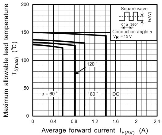
Fig. 10.4 T_{t(max)} - I_{F(AV)}
