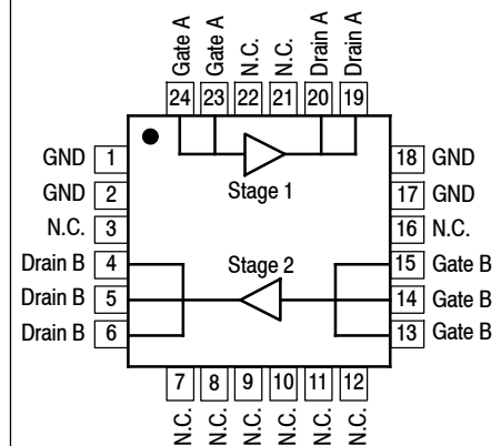
QFN 4 × 4
