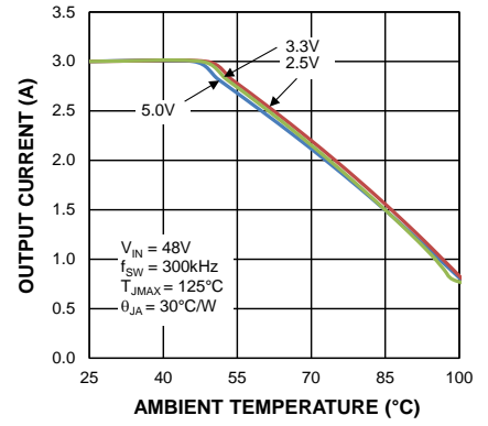
48V Input Thermal Derating MIC28511-1
