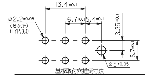
基板取付穴推奨寸法 RECOMMENDED P.C. BOARD HOLE DIMENSIONS
