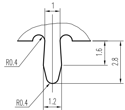
K DETAIL 2 : 1
