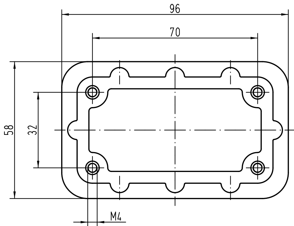
Montageausschnitt panel cut out 1:2
