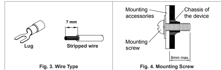
Fig. 3. Wire Type
